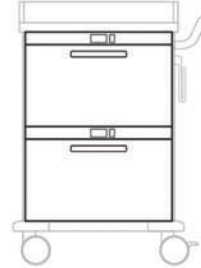
ÜRÜN KODU 543 322 830x600mm EKİPMAN (G x Y mm) Çekmeceleri ısıtmak için 2 x (600 x 375)
