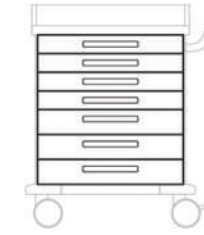
ÜRÜN KODU 543 334 830x900mm EKİPMAN (G x Y mm) 4 çekmece (600x75) 3 çekmece (600x100)
