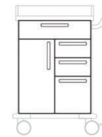
ÜRÜN KODU 543 354 980x600mm EKİPMAN (G x Y mm) 1 çekmece (600x150) 2 çekmece (300x150) 1 çekmece (300x300) 1 kanatlı kapı (300 x 600) 1 raf
