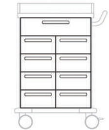
ÜRÜN KODU 543 335 980x600mm EKİPMAN (G x Y mm) 1 çekmece (600x150) 8 çekmece (300x150)
