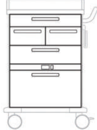
ÜRÜN KODU 543 321 830x600mm EKİPMAN (G x Y mm) 1 çekmece (600x100) 2 çekmece (300x150) 1 çekmece (600x150) Çekmeceyi ısıtmak için
