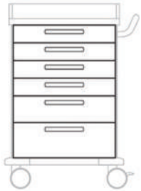
ÜRÜN KODU 543 341 830x600mm EKİPMAN (G x Y mm) 4 çekmece (600x100) 1 çekmece (600x150) 1 çekmece (600x200)
