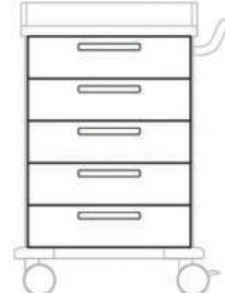
ÜRÜN KODU 543 284 830x600mm EKİPMAN (G x Y mm) 5 çekmece (600x150)
